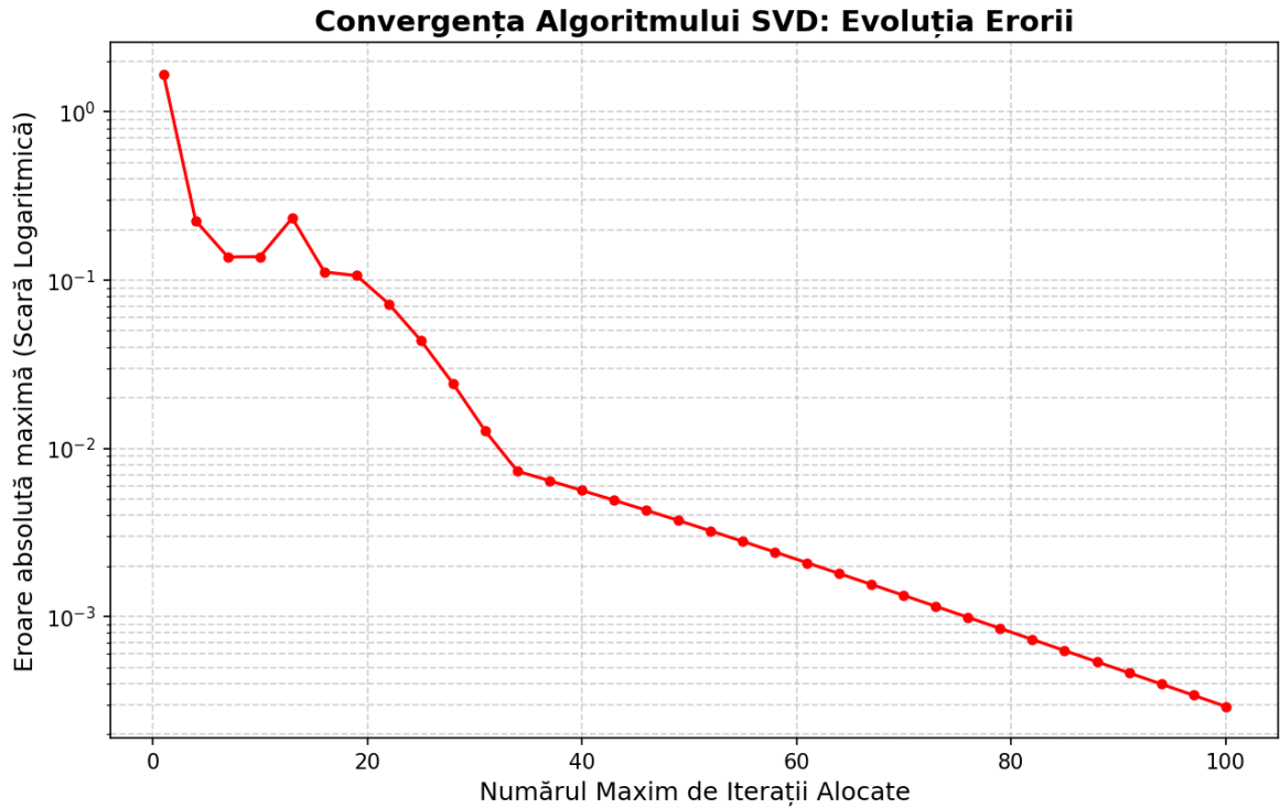
Figura 3: Graficul de evoluție a erorii
